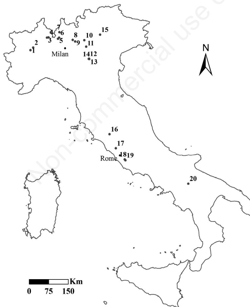
Fig. 1. Location of the lakes considered in the analysis: 1, Candia; 2, Viverone; 3, Monate; 4, Varese; 5, Alserio; 6, Segrino; 7, Como; 8, Endine; 9, Iseo; 10, Idro; 11, Garda; 12, Mantova Superiore; 13, Mantova Mezzo; 14, Mantova Inferiore; 15, Levico; 16, Bolsena; 17, Bracciano; 18, Albano; 19, Nemi; 20, Lago Grande.
